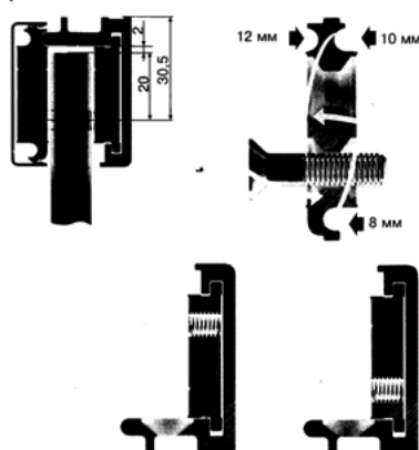
Безопасный вариант крепления стекла
