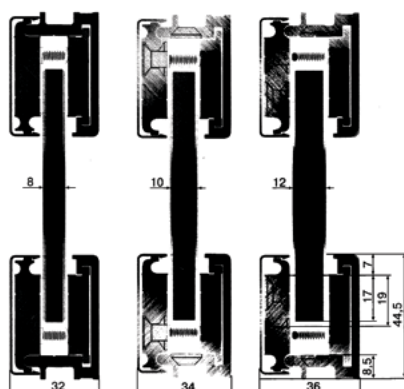
Обычный вариант крепления стекла
