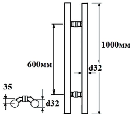
Ручка дверная двойная с отступом
