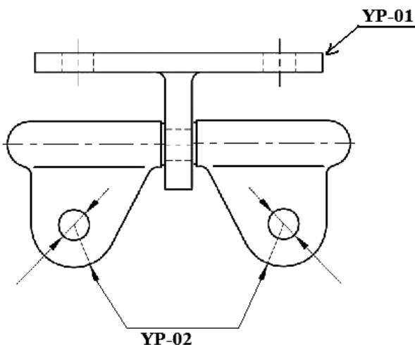
Крепление к стене двух расходящихся вант
